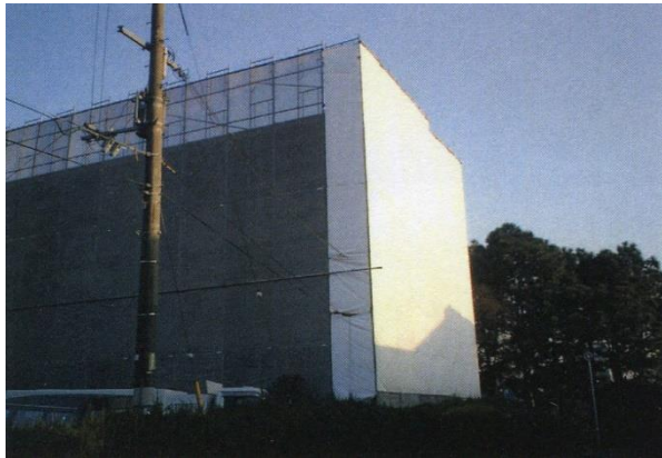
防音シート張り(隣接民家付近)
